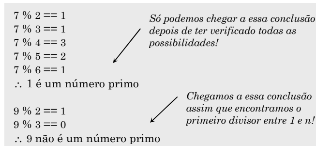
Figura 3.8 – Verificando se um número é primo
