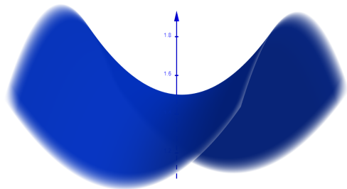
Figura: f(x) = x_1^2 - x_2^2 + \frac{3}{2} , e p = (0, 0) não é máximo nem mínimo local
