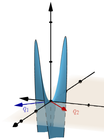
Figura: f \circ Q(y) = f(y_1 q_1 + y_2 q_2) = y_1^2 - y_2^2 ou seja o gráfico da função (não linear) f é uma rotação do gráfico de f \circ Q (a qual é uma sela de cavalo)
