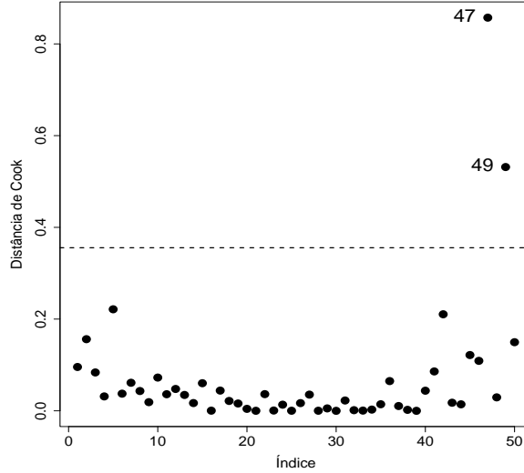
Figura 2.4: Gráfico da distância de Cook aproximada referente ao modelo gama ajustado ao dados sobre desempenho de turbinas de avião.
