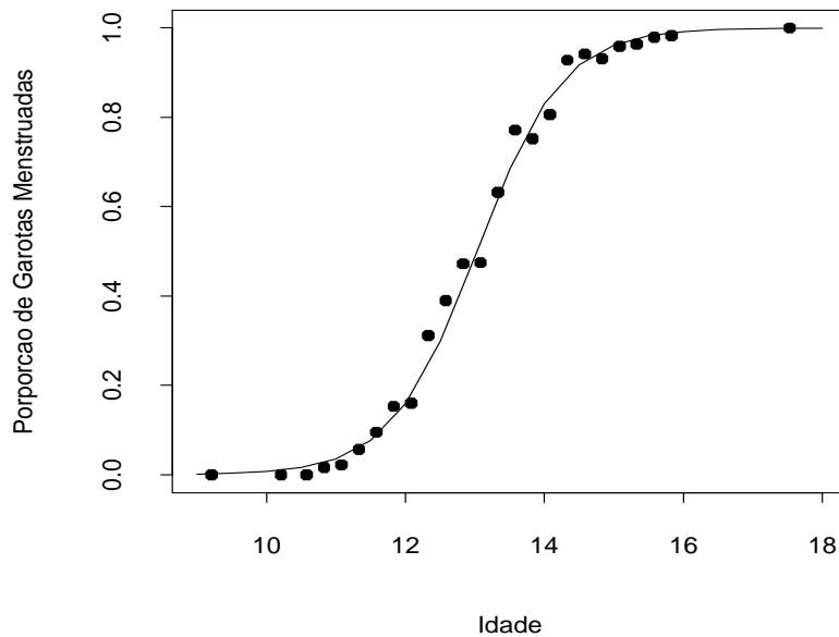
Figura 3.11: Curva ajustada pelo modelo logístico linear para a proporção de garotas de Varsóvia.
