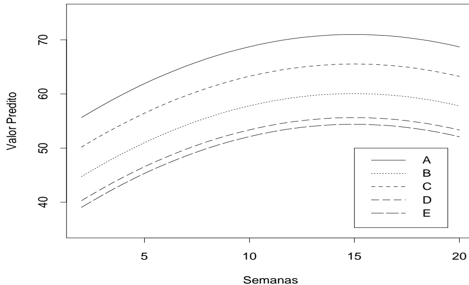
Figura 2.30: Valores preditos para a força média de cisalhamento para as 5 formas de snacks através do modelo com resposta normal inversa.
