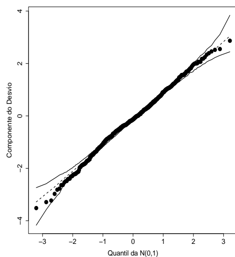
Figura 2.29: Gráfico normal de probabilidades referente ao modelo com resposta normal inversa ajustado aos dados sobre snacks .
