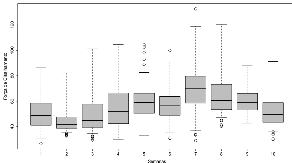
Figura 2.26: Boxplots da força de cisalhamento segundo a semana e para todos os grupos.
