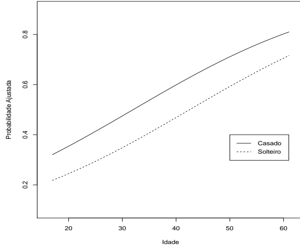
Figura 3.4: Probabilidade ajustada de preferência por caso americano segundo a idade e o estado civil do comprador.
