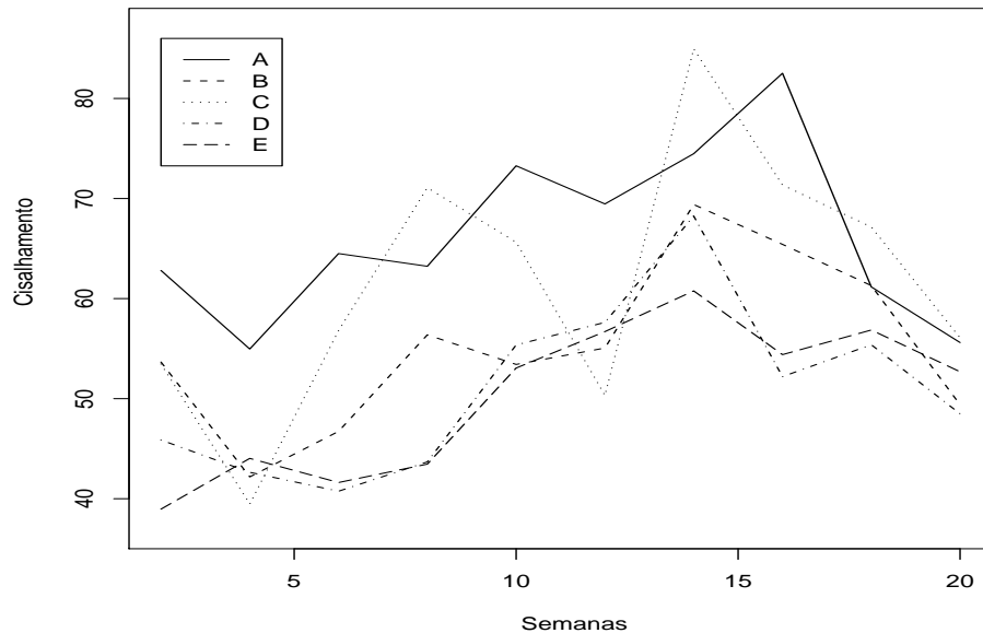
Figura 2.27: Perfis da força de cisalhamento segundo as semanas e os grupos.
