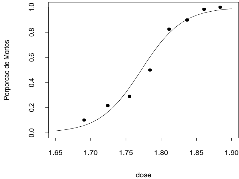
Figura 3.9: Modelo logístico ajustado à proporção de besouros mortos.
