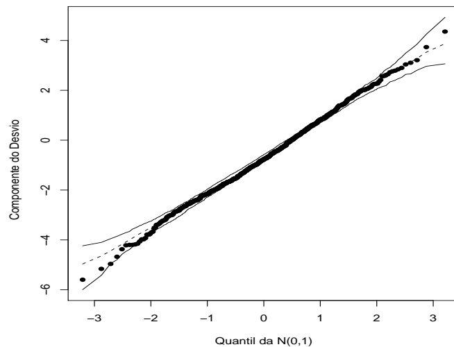
Figura 2.36: Gráfico normal de probabilidades para o resíduo componente do desvio para a dispersão referente ao MLG duplo com resposta gama ajustado aos dados sobre snacks .
