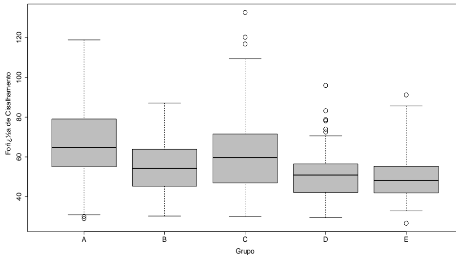
Figura 2.25: Boxplots da força de cisalhamento segundo o grupo e para todas as semanas.
