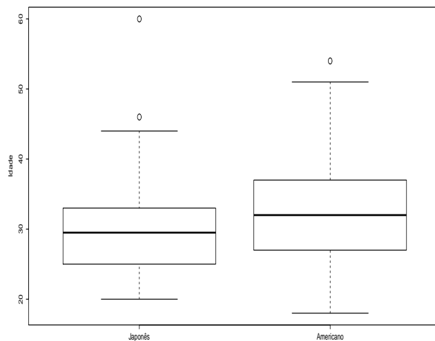
Figura 3.3: Boxplots da idade dos compradores de automóveis japonês e americano.
