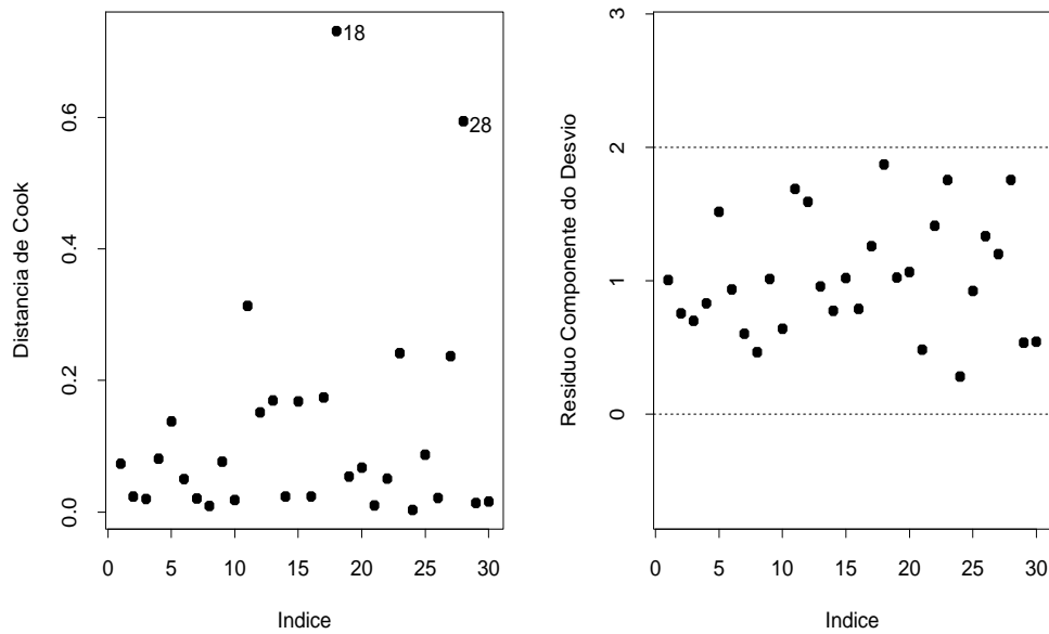
Figura 3.17: Gráficos de diagnóstico para o modelo logístico condicional aplicado aos dados sobre diabetes.
