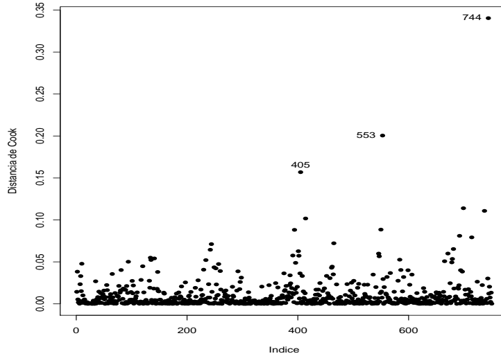
Figura 2.33: Gráfico da distância de Cook para as estimativas dos coeficientes da média referente ao MLG duplo com resposta gama ajustado aos dados sobre snacks .
