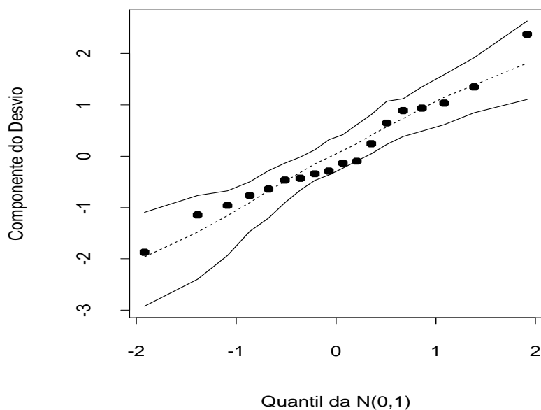
Figura 3.14: Gráfico normal de probabilidades para o resíduo corrigido para o modelo logístico de retas paralelas ajustado aos dados sobre três tipos de inseticida.
