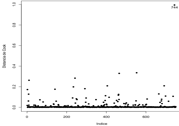
Figura 2.34: Gráfico da distância de Cook para as estimativas dos coeficientes da dispersão referente ao MLG duplo com resposta gama ajustado aos dados sobre snacks .
