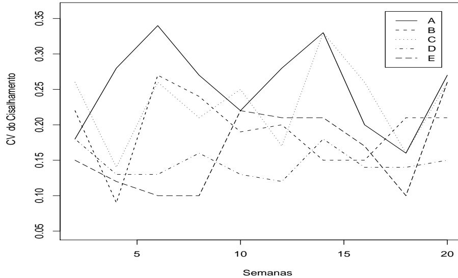
Figura 2.32: Perfis do CV da força de cisalhamento segundo as semanas e os grupos.
