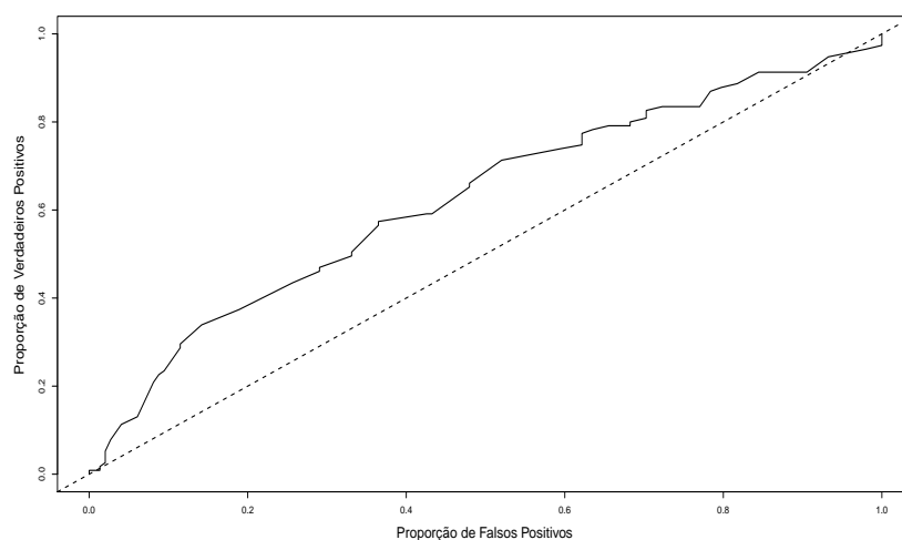
Figura 3.7: Curva ROC referente ao modelo logístico ajustado aos dados sobre preferência de consumidores.
