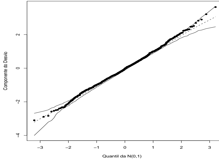
Figura 2.35: Gráfico normal de probabilidades para o resíduo componente do desvio para a média referente ao MLG duplo com resposta gama ajustado aos dados sobre snacks .
