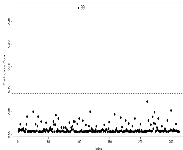
Figura 3.5: Distância de Cook referente ao modelo logístico ajustado aos dados sobre preferência de consumidores.
