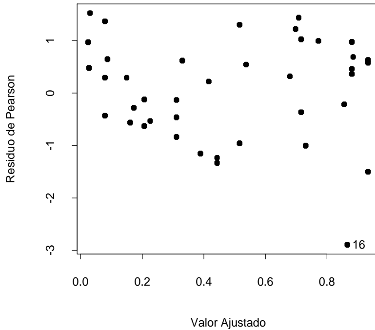
Figura 3.16: Gráfico de resíduos de Pearson contra os valores ajustados para o modelo logístico de sobredispersão ajustado aos dados sobre rotifers .
