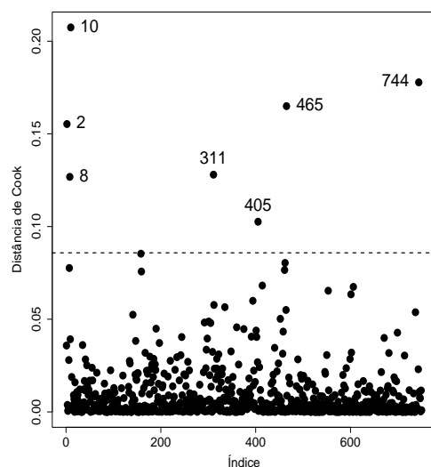
Figura 2.31: Gráfico da distância de Cook referente ao modelo com resposta normal inversa ajustado aos dados sobre snacks .
