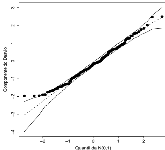
Figura 2.16: Gráfico normal de probabilidades referente ao modelo gama ajustado aos dados sobre espínhel de fundo.
