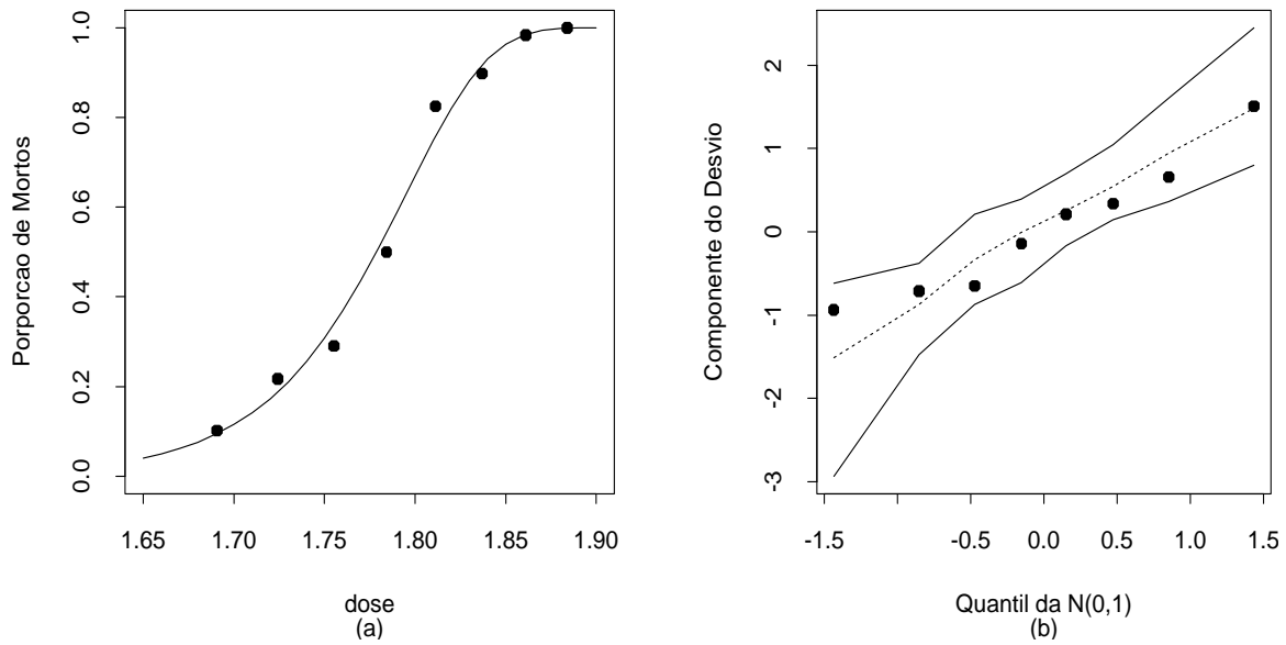
Figura 3.10: Curva ajustada para a proporção de besouros mortos (a) e gráfico normal de probabilidades sob o modelo complementar log-log (b).
