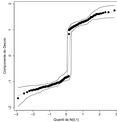
Figura 3.6: Gráfico normal de probabilidades para o resíduo componente do desvio referente ao modelo logístico ajustado aos dados sobre preferência de consumidores.
