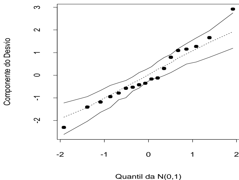
Figura 3.13: Gráfico normal de probabilidades para o modelo logístico de retas paralelas ajustado aos dados sobre três tipos de inseticida.
