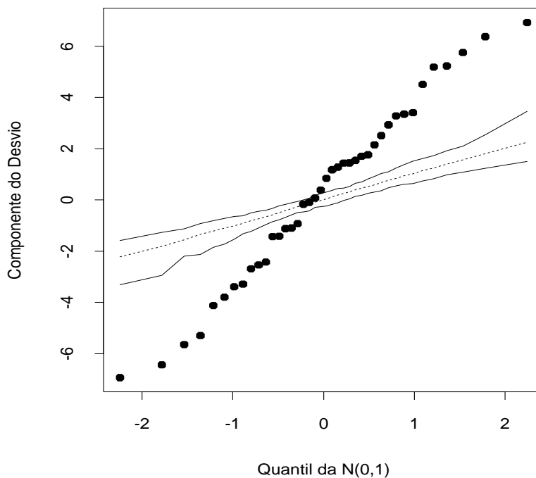
Figura 3.15: Gráfico normal de probabilidades do modelo logístico ajustado aos dados sobre rotifers .
