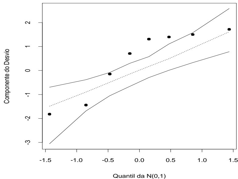
Figura 3.8: Gráfico normal de probabilidades referente ao modelo logístico ajustado aos dados sobre exposição de besouros.
