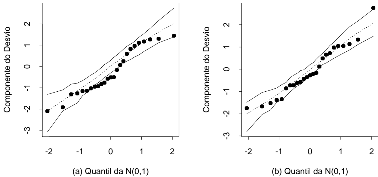
Figura 3.12: Gráficos normais de probabilidades para os modelos logístico com componente sistemática linear (a) e não linear (b) ajustados aos dados sobre garotas de Varsóvia.
