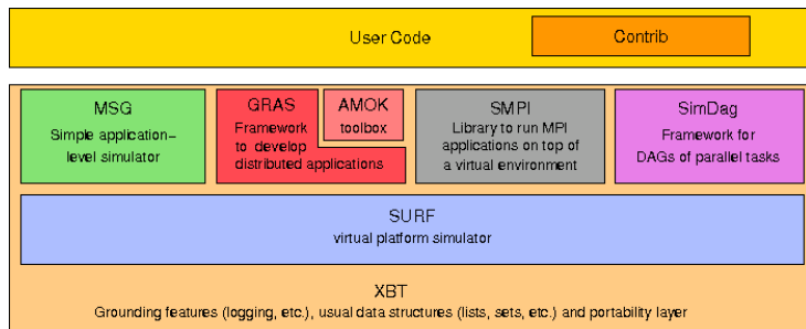
Figura: Módulos do SimGrid
