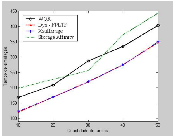
Figura: Comparação dos algoritmos
