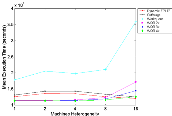
Figura: Comparação dos algoritmos
