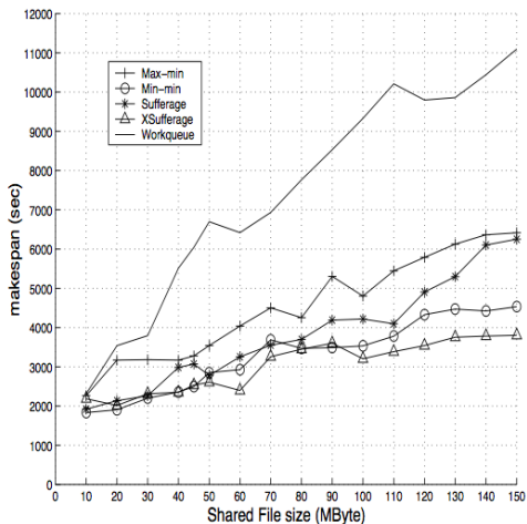
Figura: Comparação dos algoritmos
