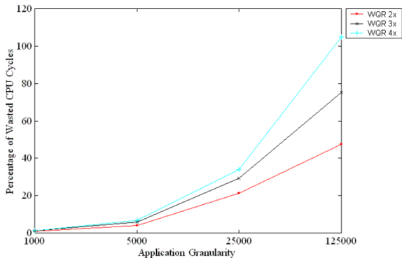
Figura: Comparação dos algoritmos
