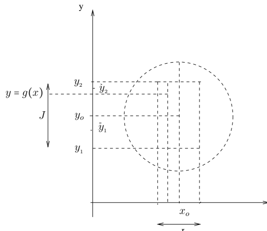
Figura 3: Teorema 1 das Funções Implícitas
