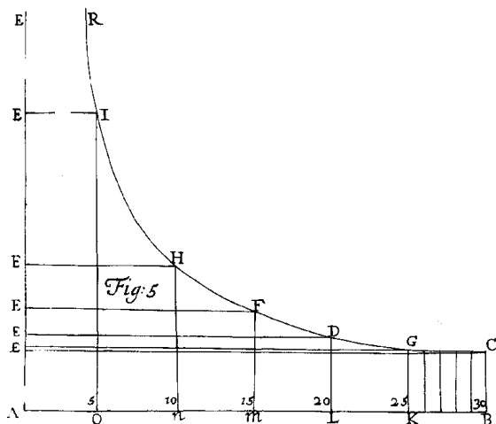
Função contínua de Halley
