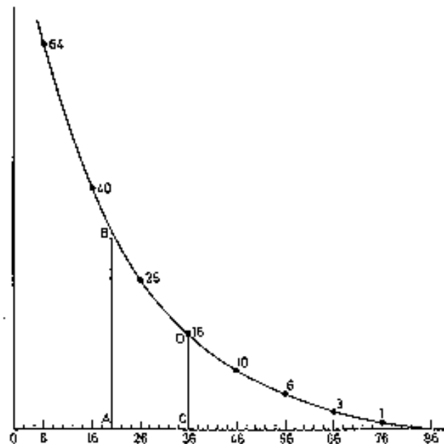
Espectativa de vida de Christiaan Huygens (1669)
