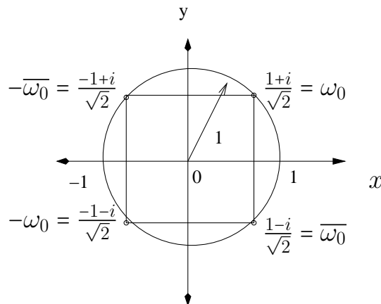
Figura 1: As quatro raízes quartas de z = -1 .
